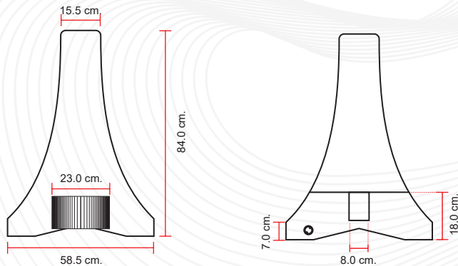
VISTA LATERAL
