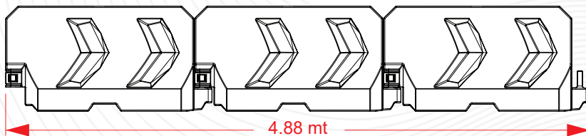
EJEMPLO 3 BARRERAS ENGANCHADAS
