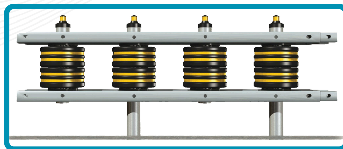
Roll Defender Doble para vías de alta velocidad
